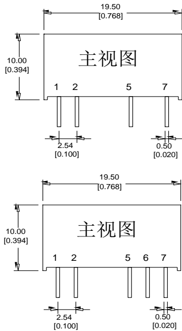
封装尺寸图
