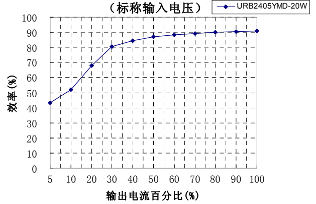
效率VS输出负载曲线图
