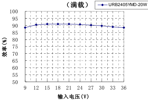
效率VS输入电压曲线图
