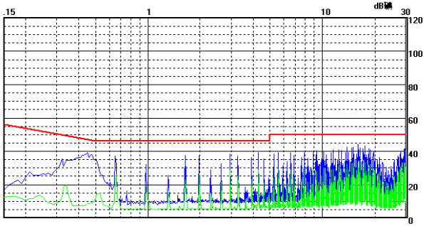
URB2405YMD-20W 传导骚扰 Class B 测试效果图（正线）
