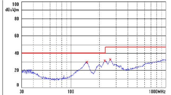
URB2405YMD-20W 辐射骚扰 Class B 测试效果图（水平）
