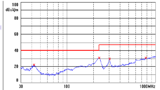
URB4815YMD-20W 辐射骚扰 Class B 测试效果图（水平）
