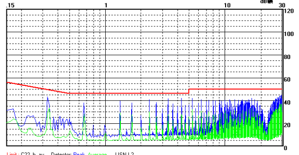
URB4815YMD-20W 传导骚扰 Class B 测试效果图（负线）
