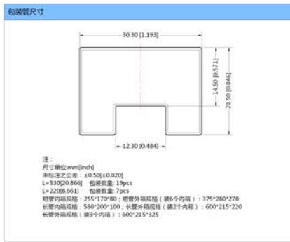
卧式封装（不带散热片）
