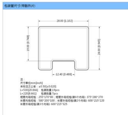
卧式封装（带散热片）
