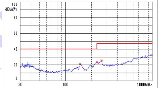
URB2405YMD-20W 辐射骚扰 Class B 测试效果图（垂直）
