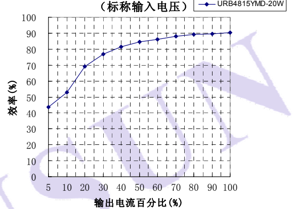
效率VS输出负载曲线图
