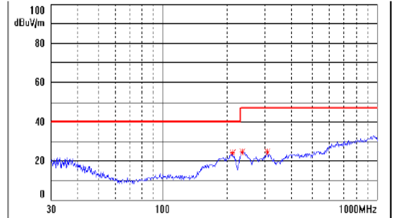
URB4815YMD-20W 辐射骚扰 Class B 测试效果图（垂直）
