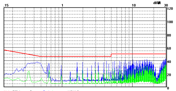
URB2405YMD-20W 传导骚扰 Class B 测试效果图（负线）
