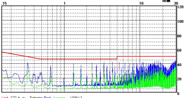
URB4815YMD-20W 传导骚扰 Class B 测试效果图（正线）
