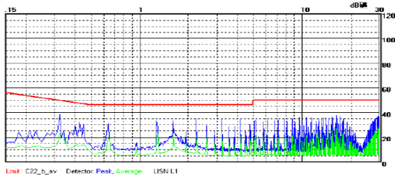
URF2405LP-20W 传导骚扰 Class B 测试效果图（正线）
