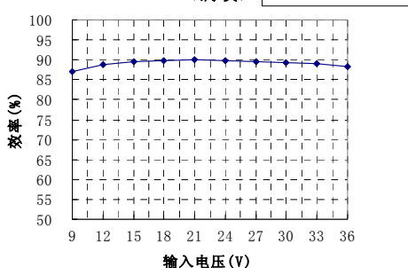
效率VS输入电压曲线图 (满载)
