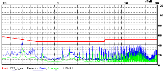
URF4815LP-20W 传导骚扰 Class B 测试效果图（正线）
