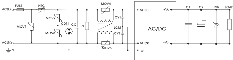
图 2 (输出外接电路同上述典型应用电路)
