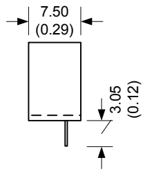
SIP4 – PLASTIC CASE
